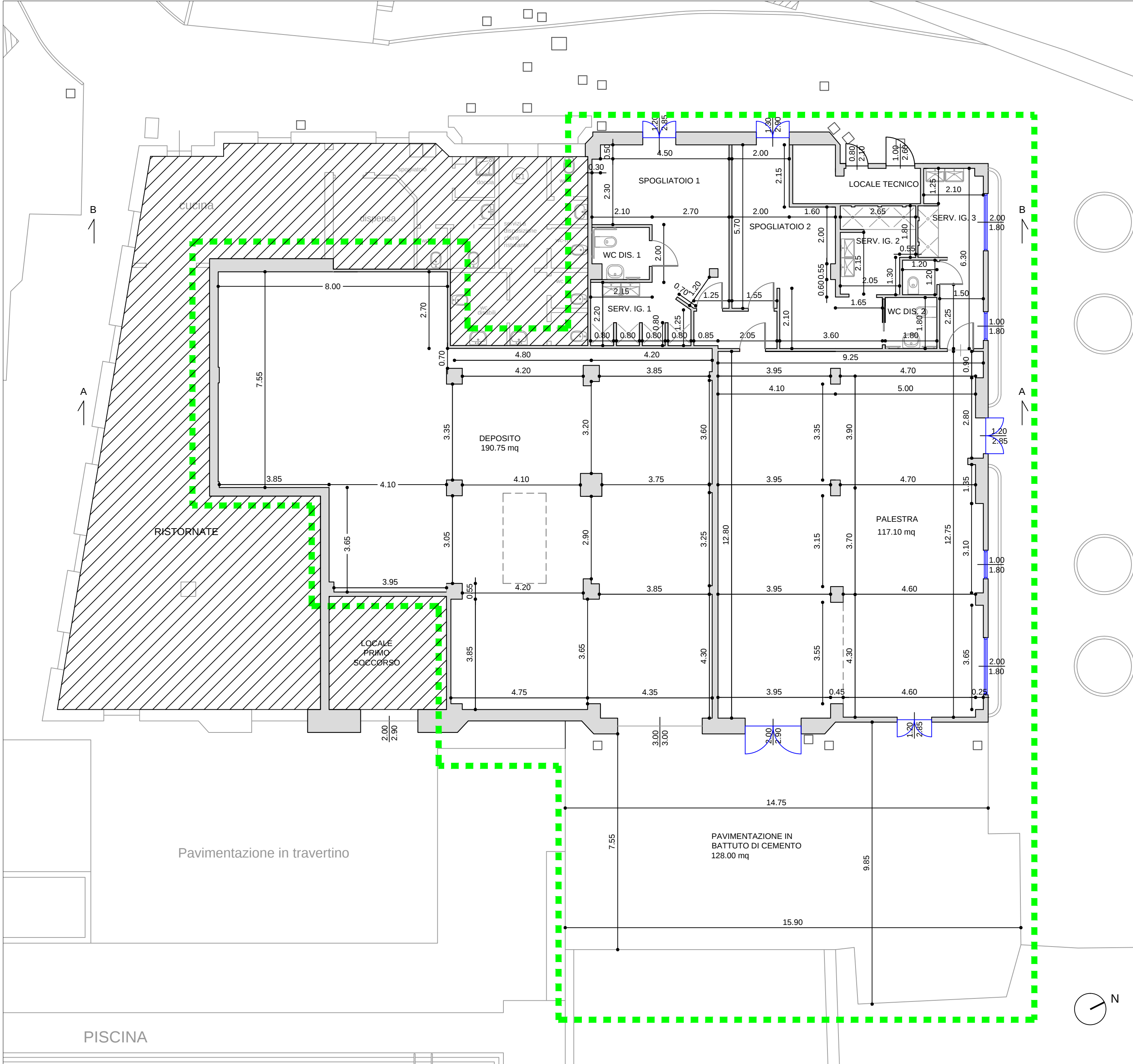
PIANTA POST OPERAM QUOTATA Scala 1:100
