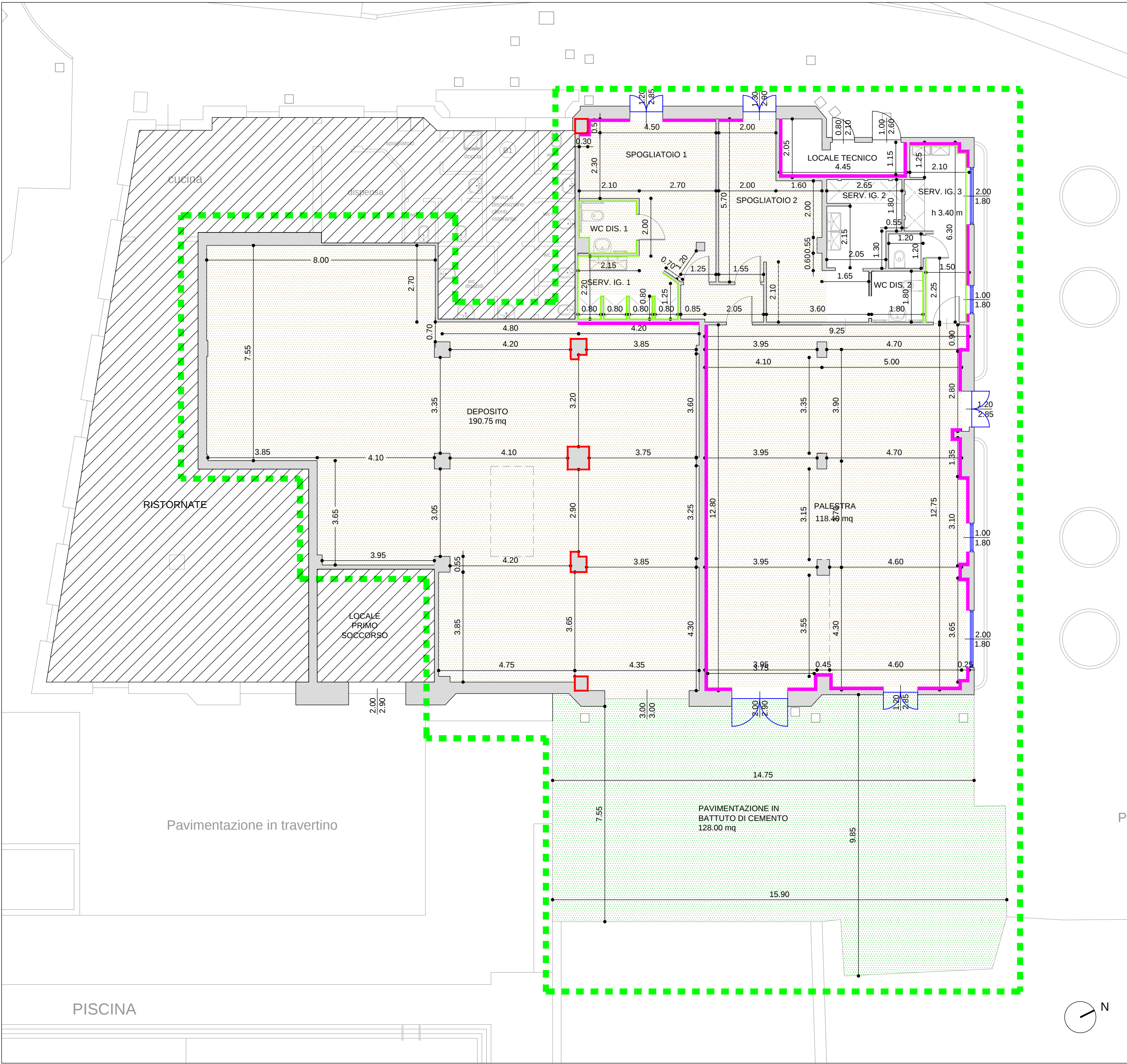
PIANTA PIANTO TERRA Scala 1:100
