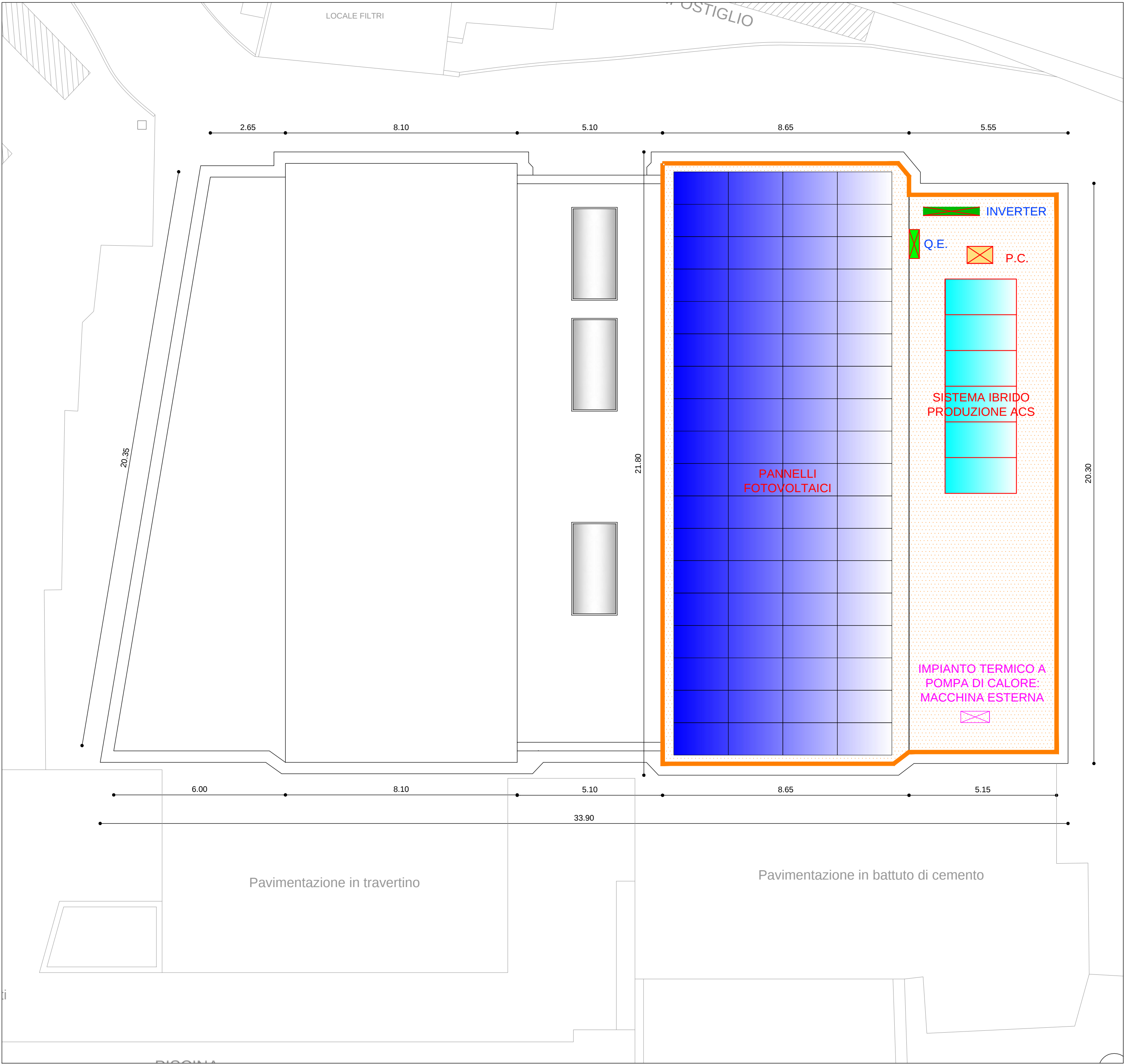
PIANTA DELLE COPERTURE Scala 1:100
