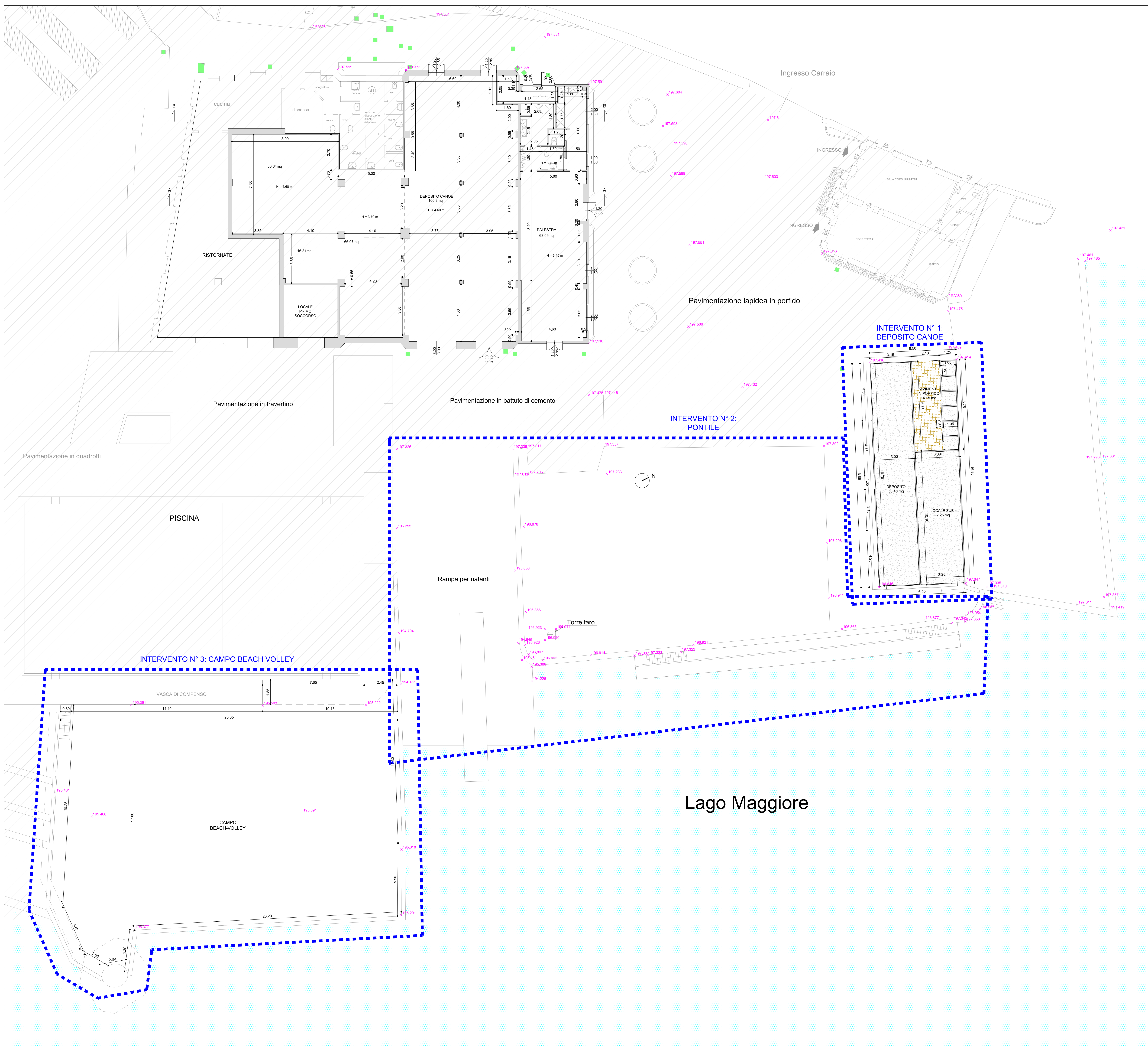
PLANIMETRIA GENERALE: STATO DEI LUOGHI Scala 1:100
