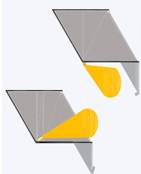
Tipo C integrata alle protezioni
