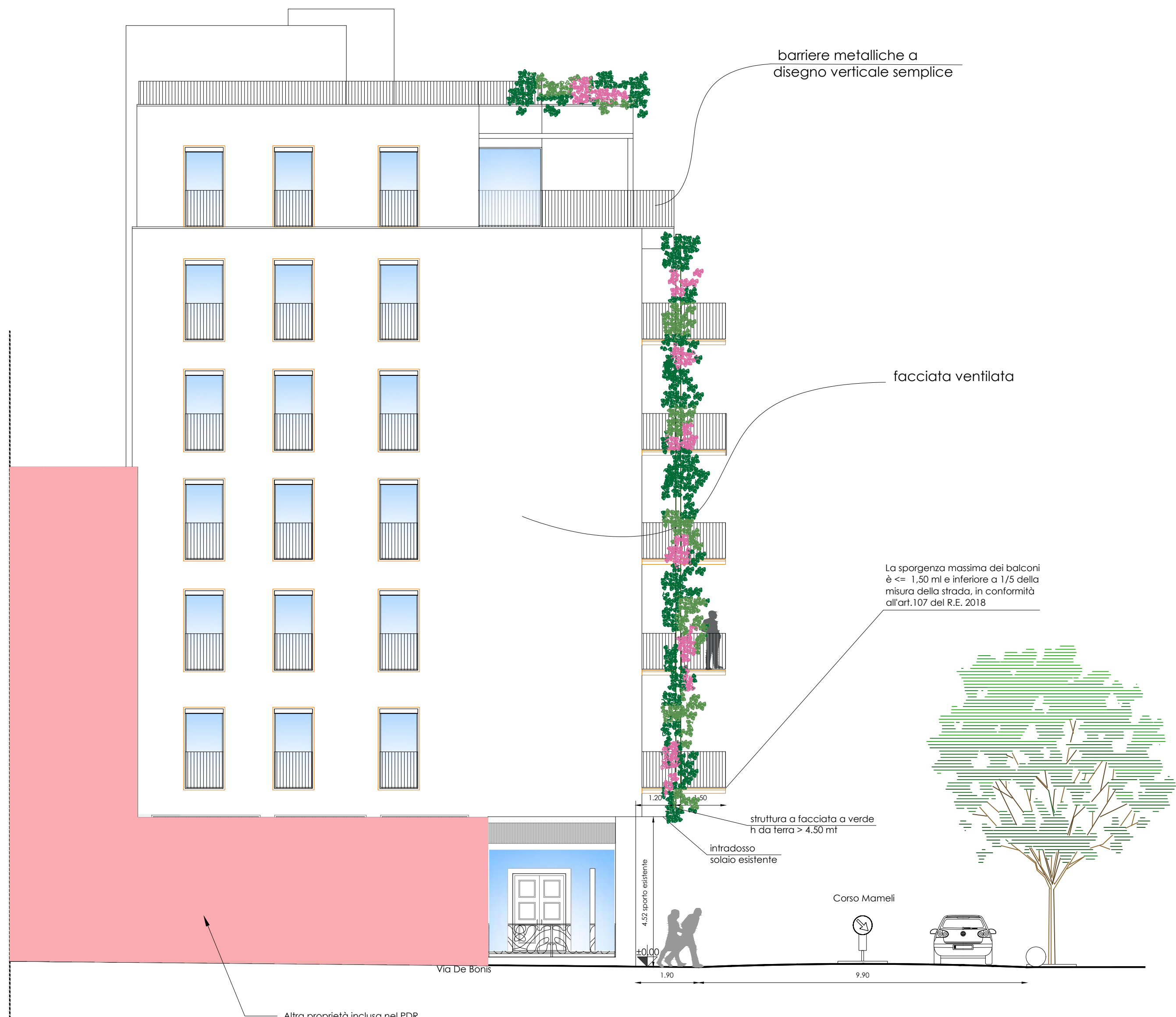
PROSPETTO SUD OVEST su Via De Bonis
